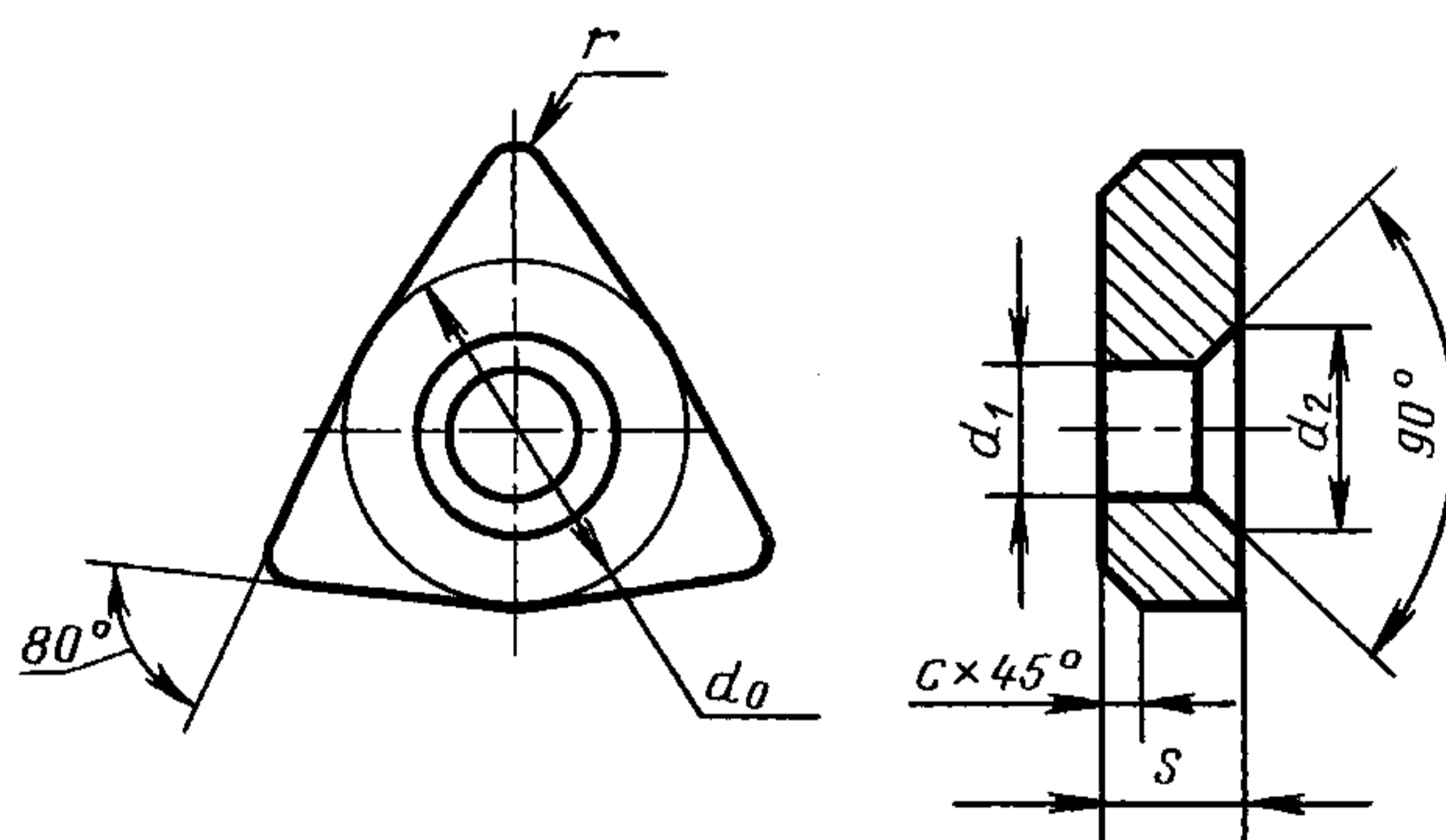
Размеры, мм
